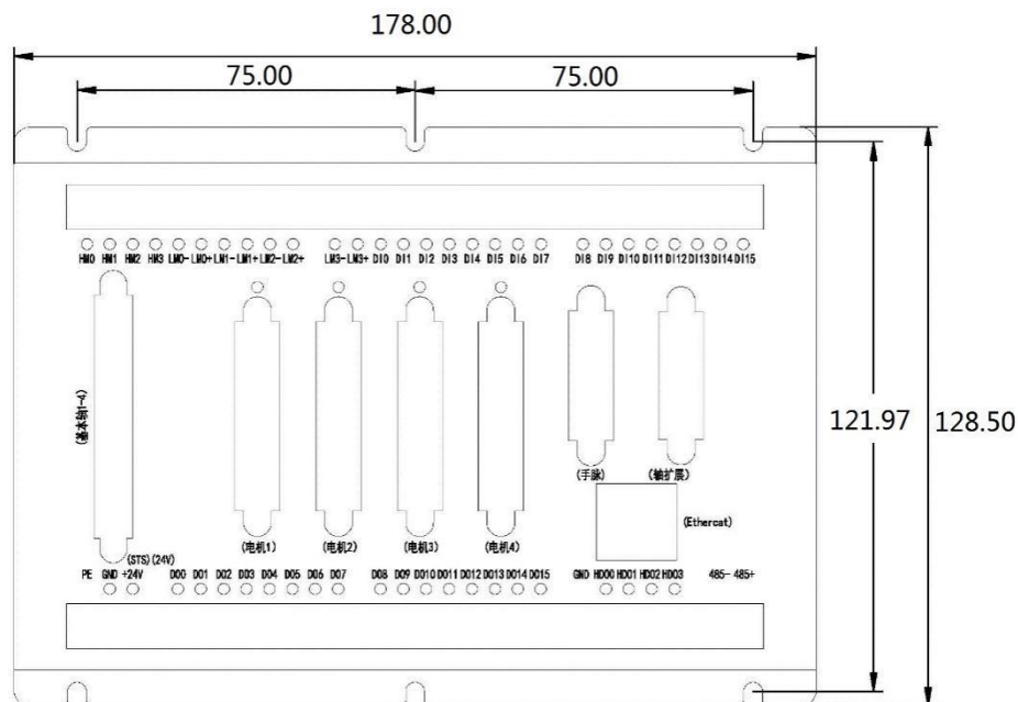
图 1.2.2 GC400A-PCIE 控制卡端子板外观及尺寸图
