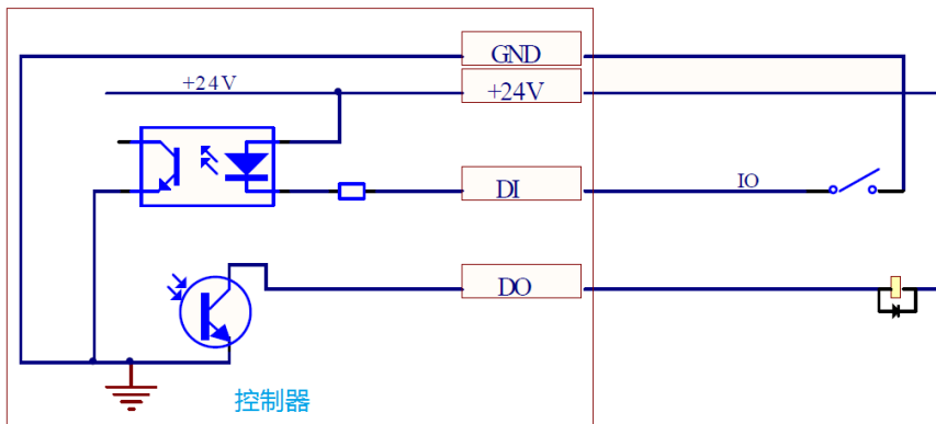
图 3.5.1 数字输入输出配线示意图
