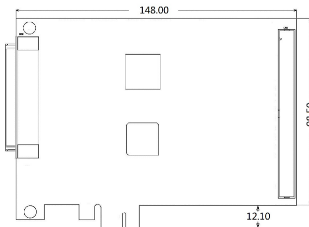
图 1.2.1 GC400A-PCIE 控制卡主卡外观及尺寸图
