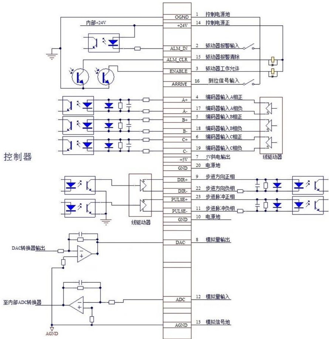
图 3.2.1 电机轴配线示意图
