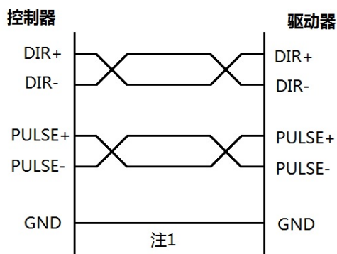
图 3.2.3 脉冲输出差分接法示意图
